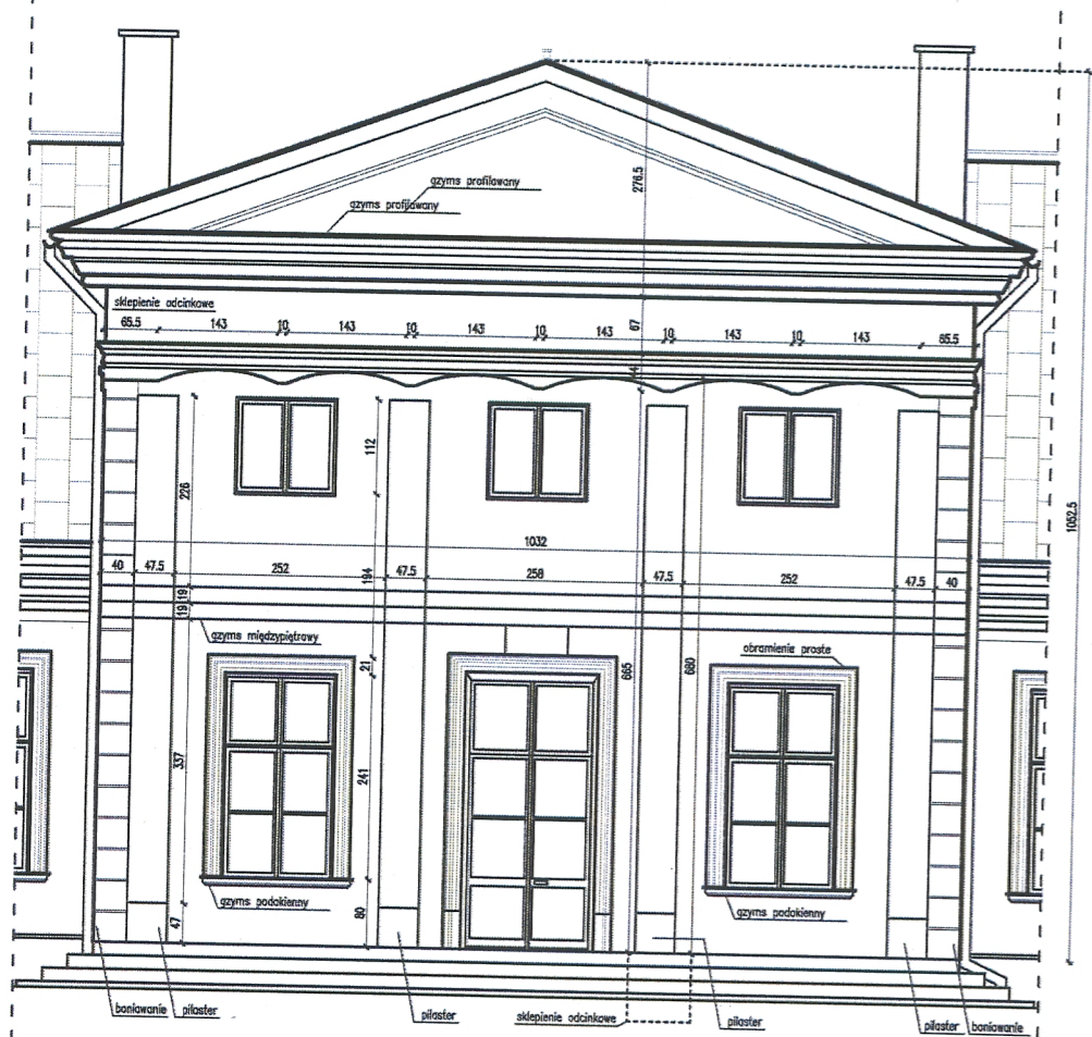
ELEWACJA PÓŁNOCNA - FRONTOWA WIDOK BEZPOŚREDNI - BEZ PORTYKU skala 1:100
