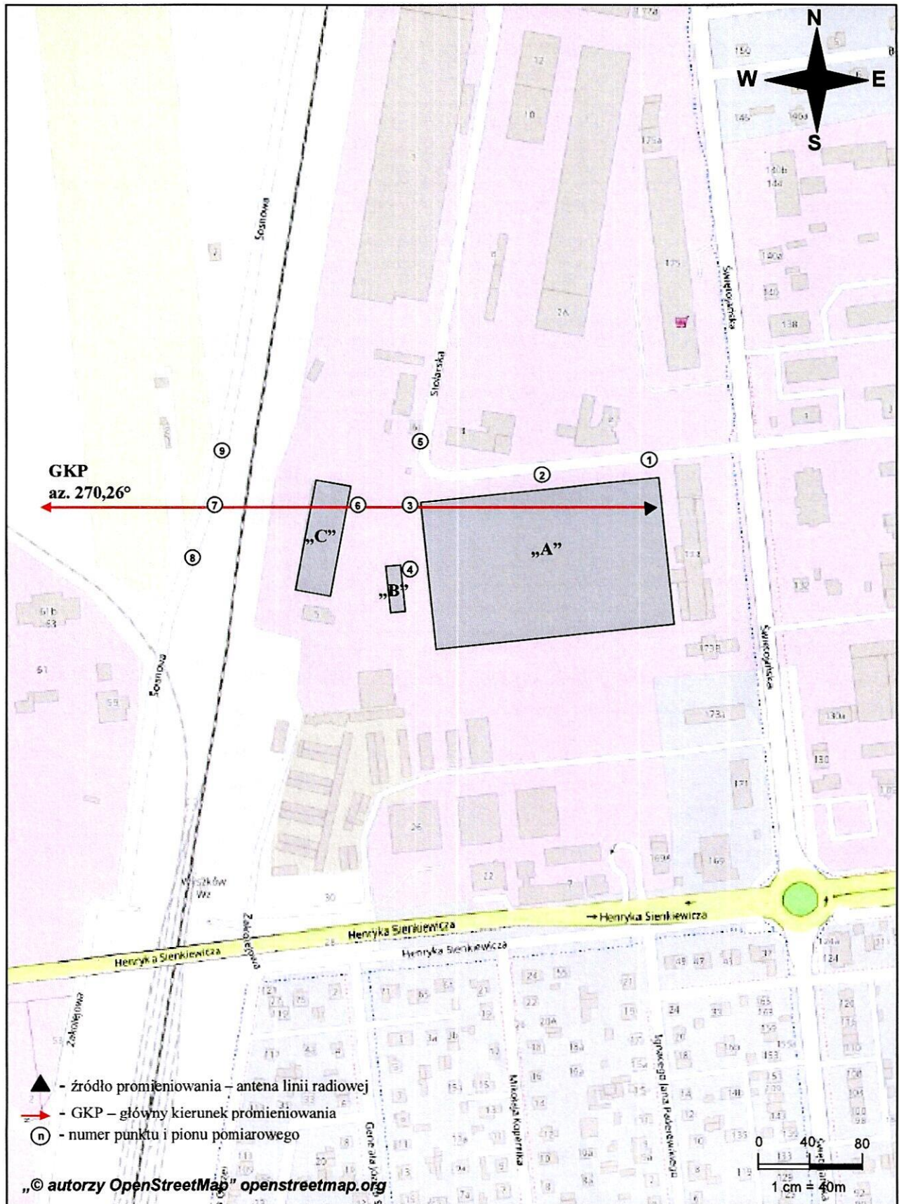
Rys. 1. Usytuowanie punktów i pionów pomiarowych w otoczeniu instalacji radiokomunikacyjnej Stacja Netia WYSWB033-WYSWM00005 Wyszków, ul. Stolarska 1
