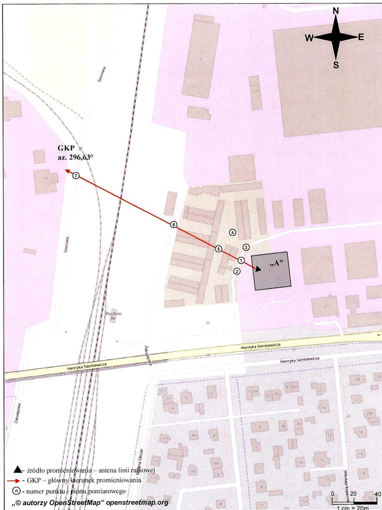
Rys. 1. Usytuowanie punktów i pionów pomiarowych w otoczeniu instalacji radiokomunikacyjnej Stacja Netia WYSWB051-WYSWM00007 Wyszków, ul. Henryka Sienkiewicza 26
